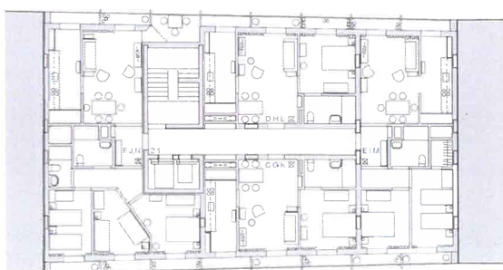
E. Planta do Piso tipo - Pisos 2-4 ESC: 1/200
