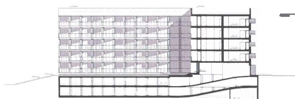
CORTE A - CORTE ALÇADO LOGRADOURO SUL-NASCENTE
