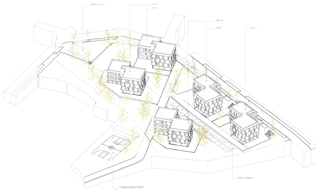
Axonometria do conjunto
