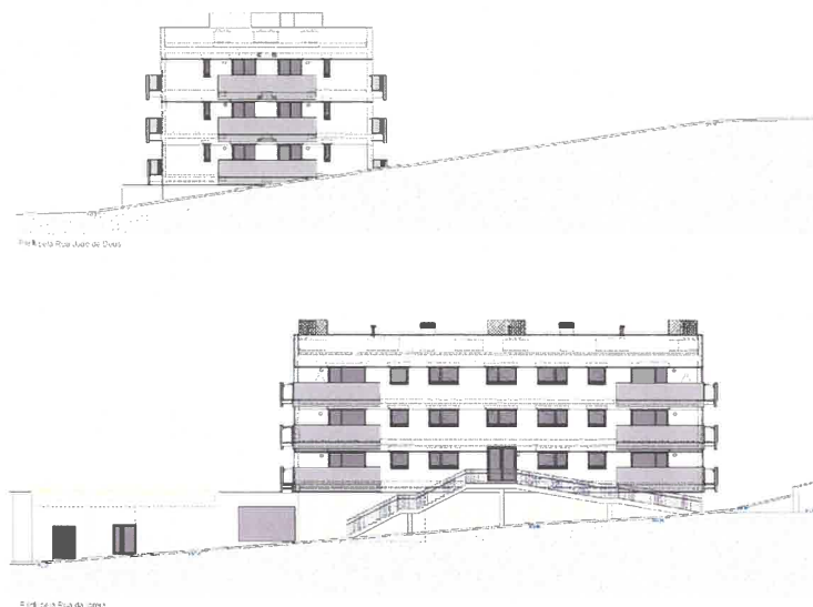
Perfis / Alçados – Empreendimento Rua da Igreja, Pedrouços (12 fogos)
