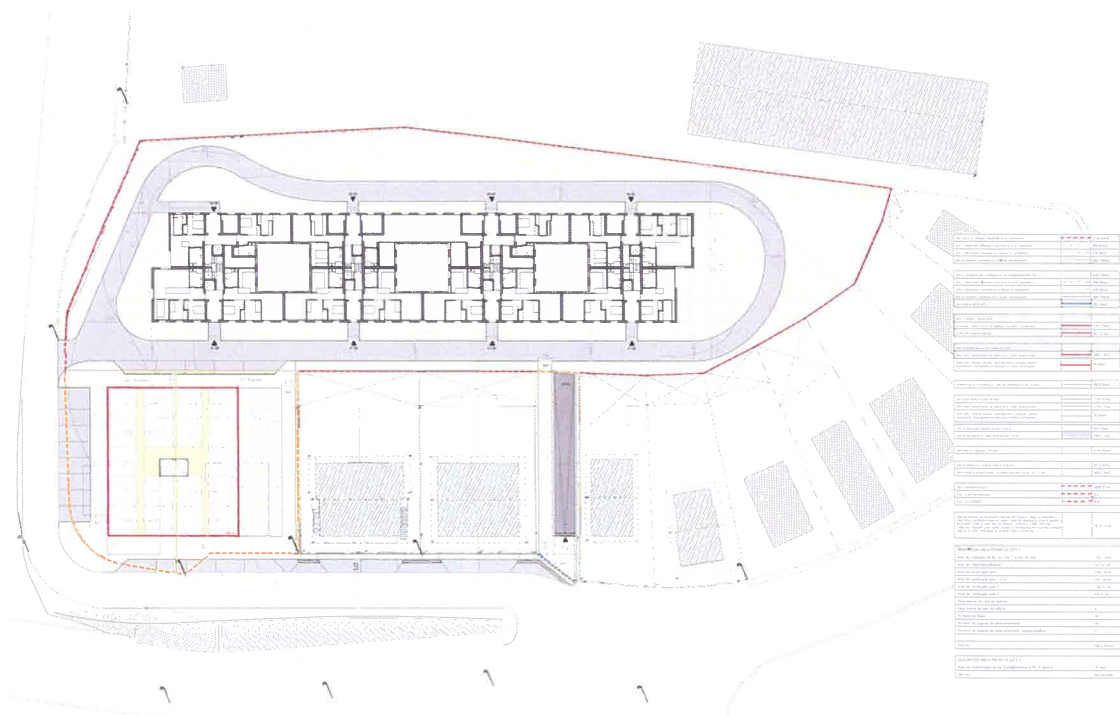
Planta de Implantação – Empreendimento Rua Prof. Oliveira Andrade, Moreira (38 fogos)
